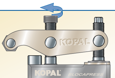
Réglage d'approche avec la molette Ø 24 ou la clé 6 pans de 5 mm
